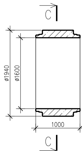
PRZEKRÓJ
