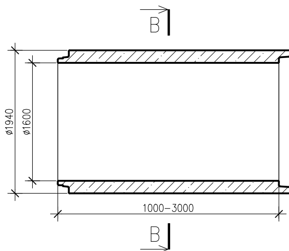
PRZEKRÓJ
